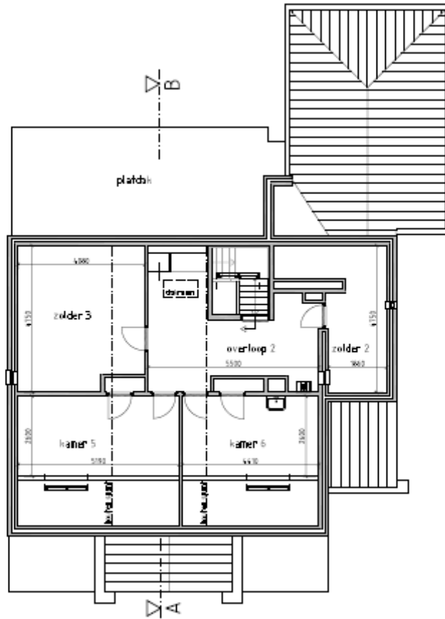
2e VERDIEPING
