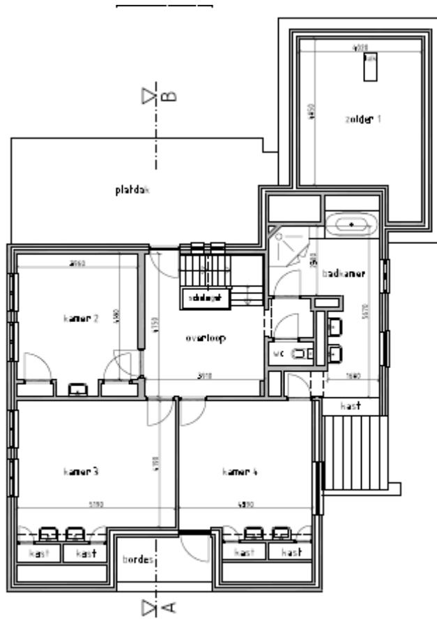
1 ste VERDIEPING
