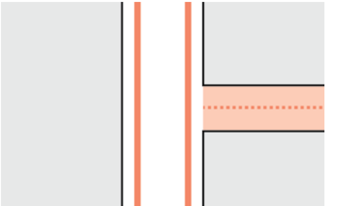
Op de kruising met stegen De doorlopende banden lopen parallel aan de gevels en zijn onafhankelijk van de stegen. De bestrating van de stegen, samen met de centrale goot, stopt bij de kruising met het trottoir van de straat.
